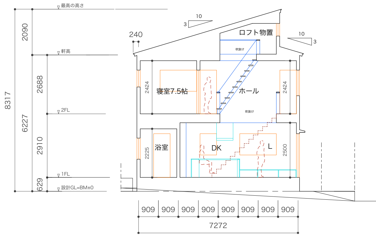
A - A' 断面図 1/100
