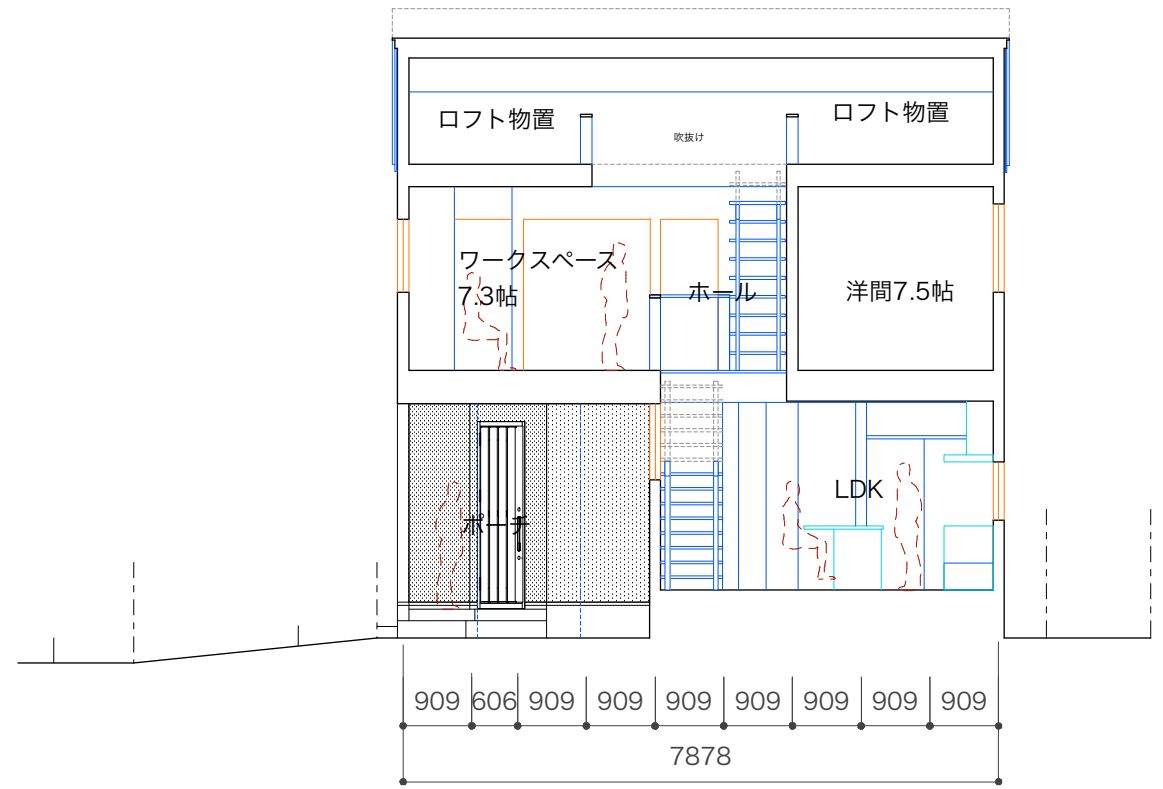
B - B' 断面図 1/100
