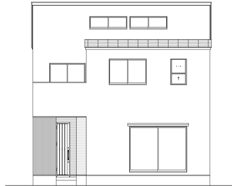
南 立面図 1/100
