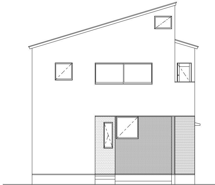
西 立面図 1/100
