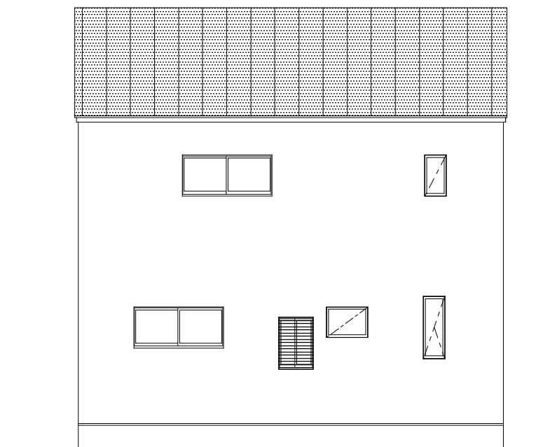
北 立面図 1/100
