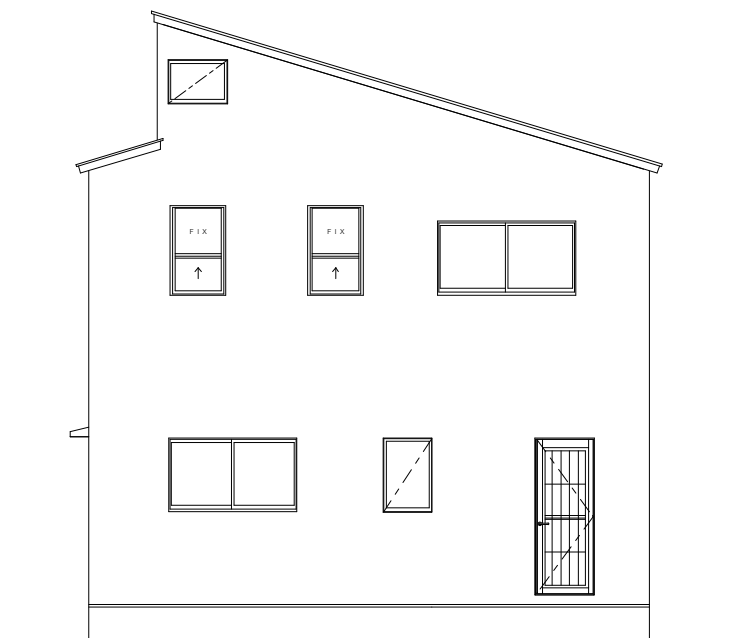
東 立面図 1/100
