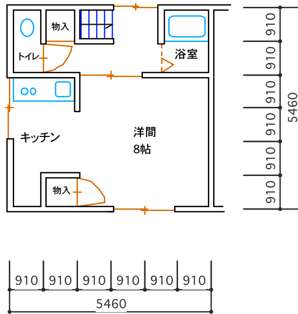
2階平面図 1/100
