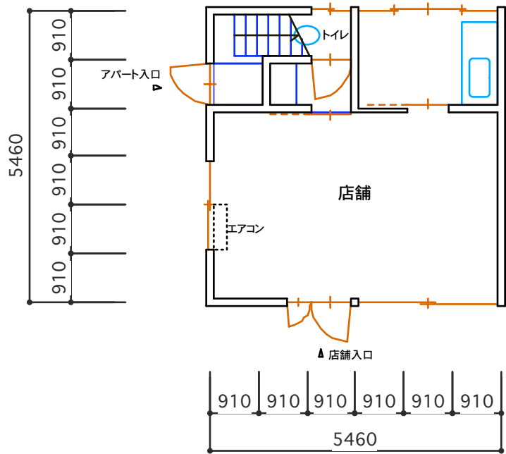
1階平面図 1/100
